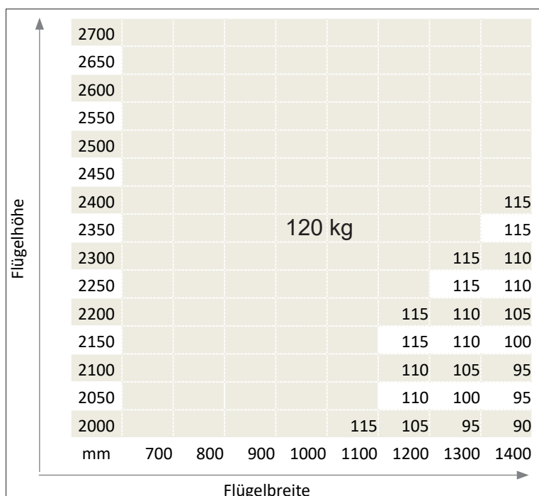
Maximal zulässige Türflügelgewichte VL-Band AL
